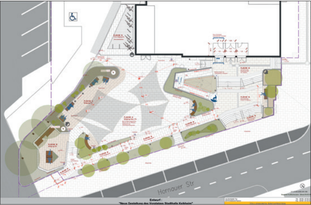
So hat das Kelkheimer Architekturbüro Gillenkirch den Vorplatz der Stadthalle gestaltet. In dem Entwurf, der Barrierefreiheit für Rollator- wie Rollstuhlfahrer garantiert, gibt es viele Grünflächen, fließende Übergänge und Platz für Autoshow's im Rahmen von Messen oder Flohmarktständen. Foto: gillenkirch-architekten
